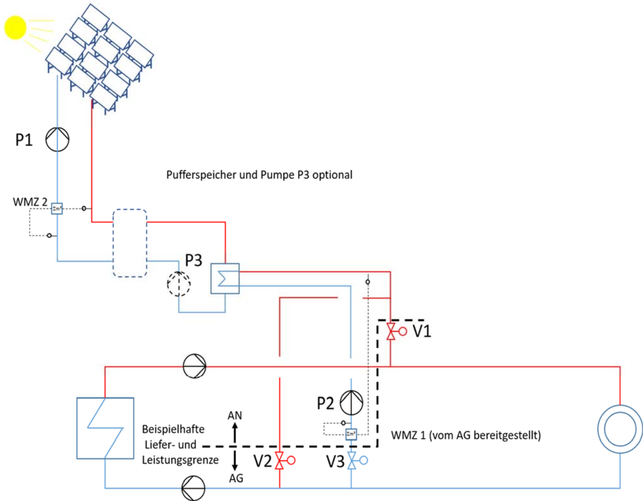
Beispielhaftes Konzept zur Einbindung der Solarthermieranlage (Schema und Liefer- und Leistungsgrenzen müssen entsprechend angepasst werden)
